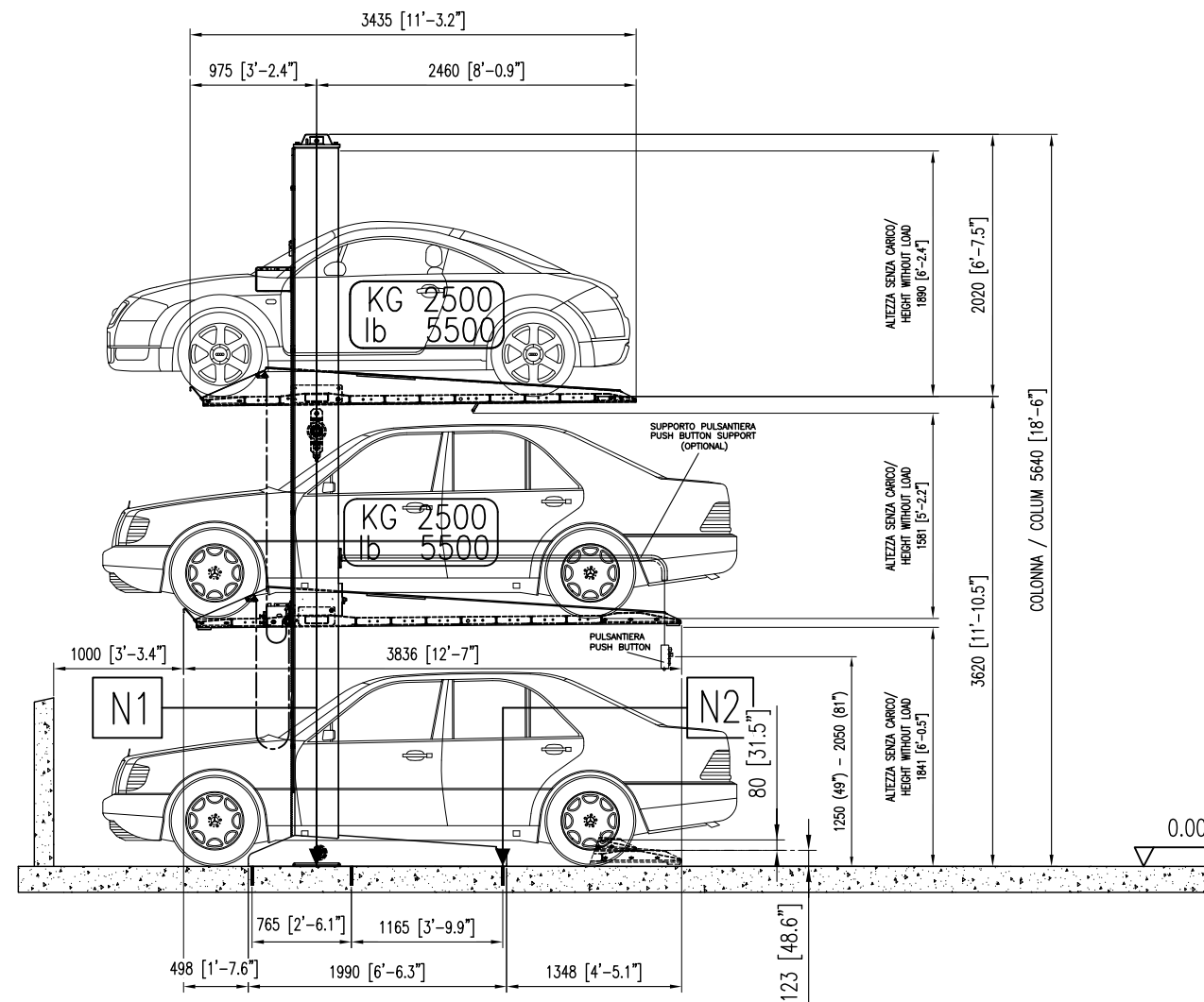
SEZIONE / SECTION
